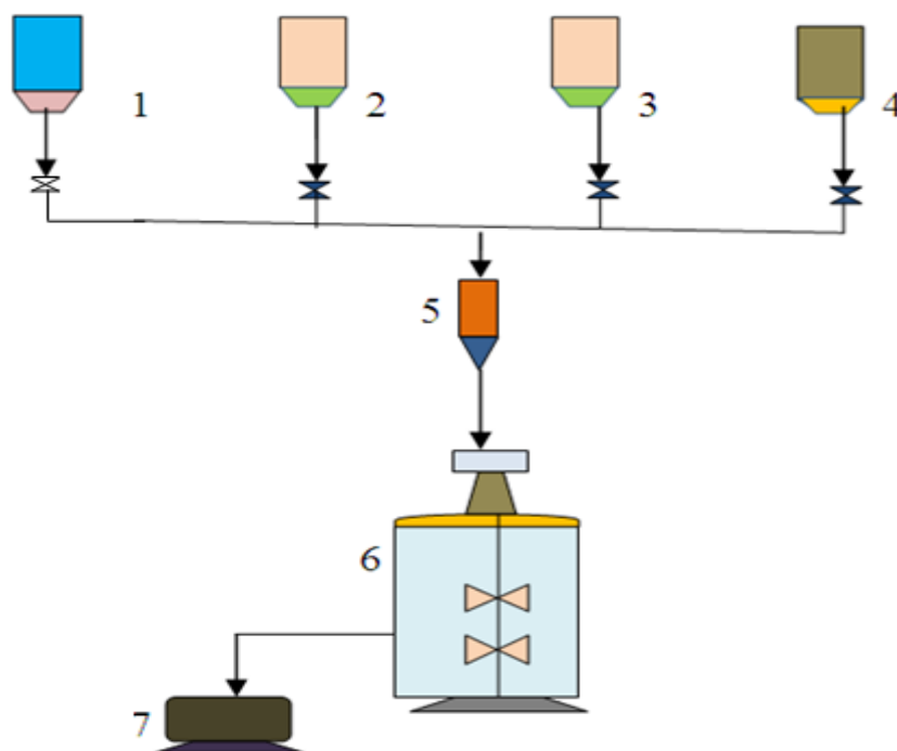
Рисунок 1. Принципиальная технологическая схема получения реагента «ЭЖКГ»:
